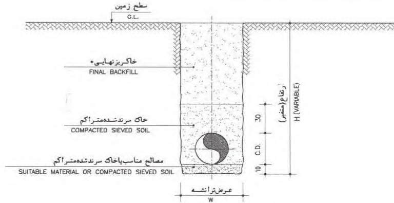
مقطع ترانشه TRENCH SECTION N.T.S
